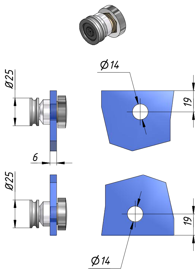
Ролик RL-19 (для KUBELE 19)
