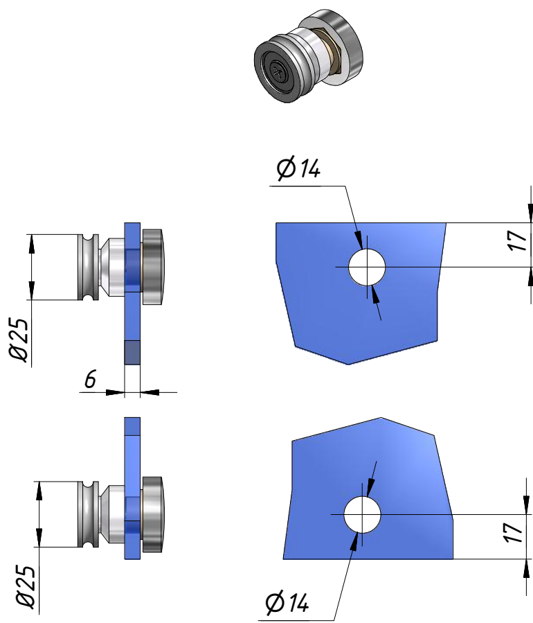
Ролик RL-19 (для GUWER)
